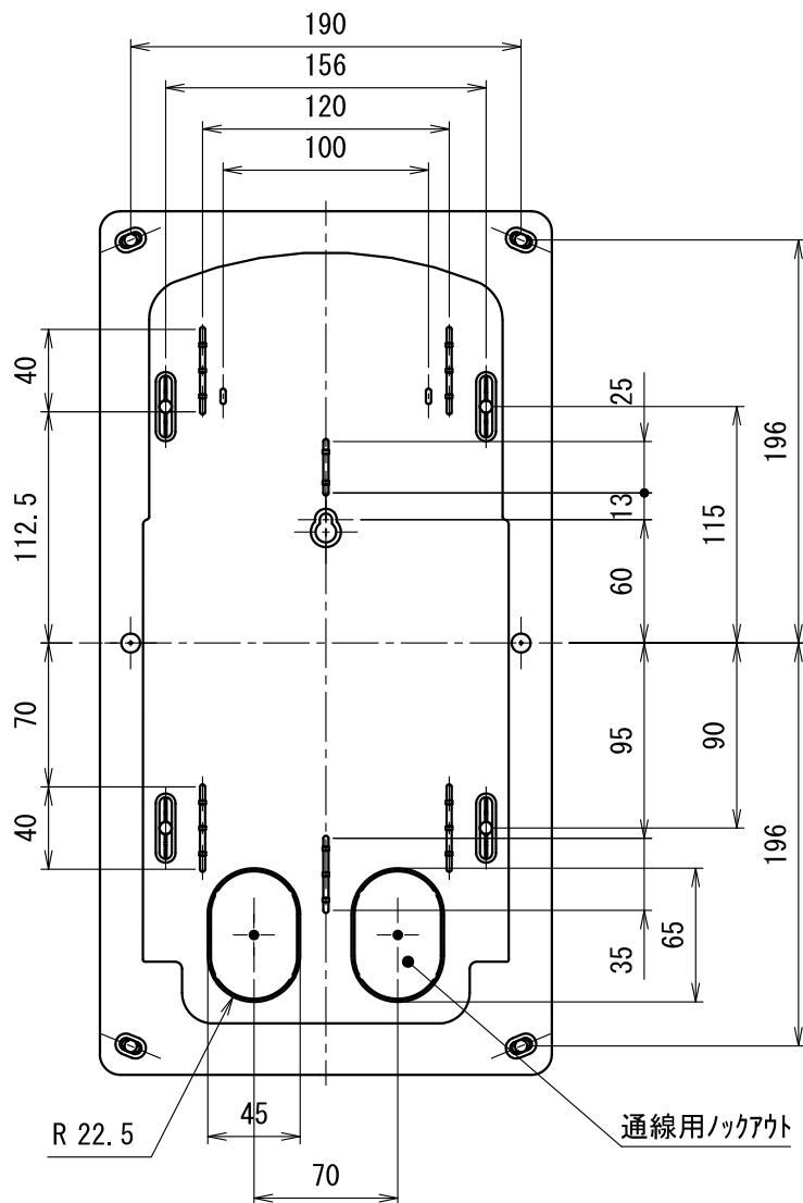
差込通線用ノックアウト (VE22用) × 2個 差込通線用ノックアウト (VE22用)
