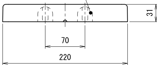
差込通線用ノックアウト (VE22用) × 2個 差込通線用ノックアウト (VE22用)
